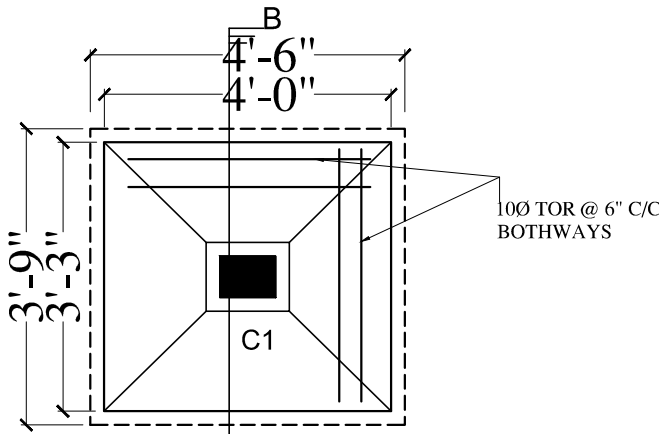
DETAIL OF FOUNDATION F1
